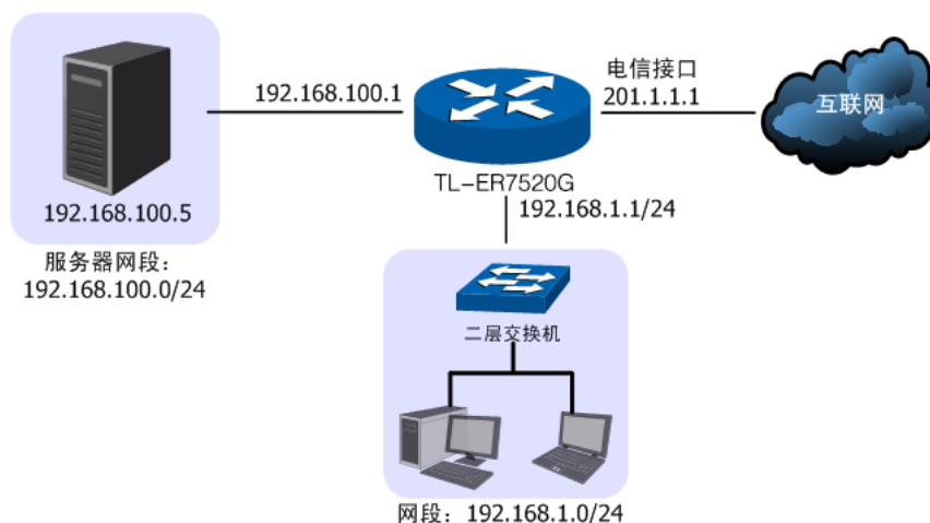
图 7-14 虚拟服务器功能组网应用
