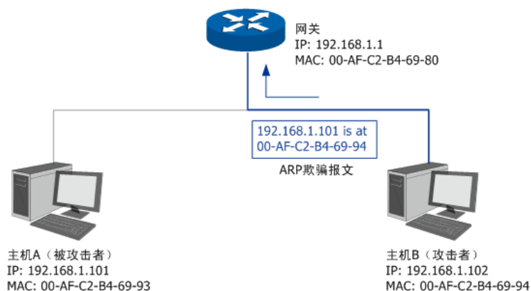
图 8-4 ARP欺骗-欺骗网关
