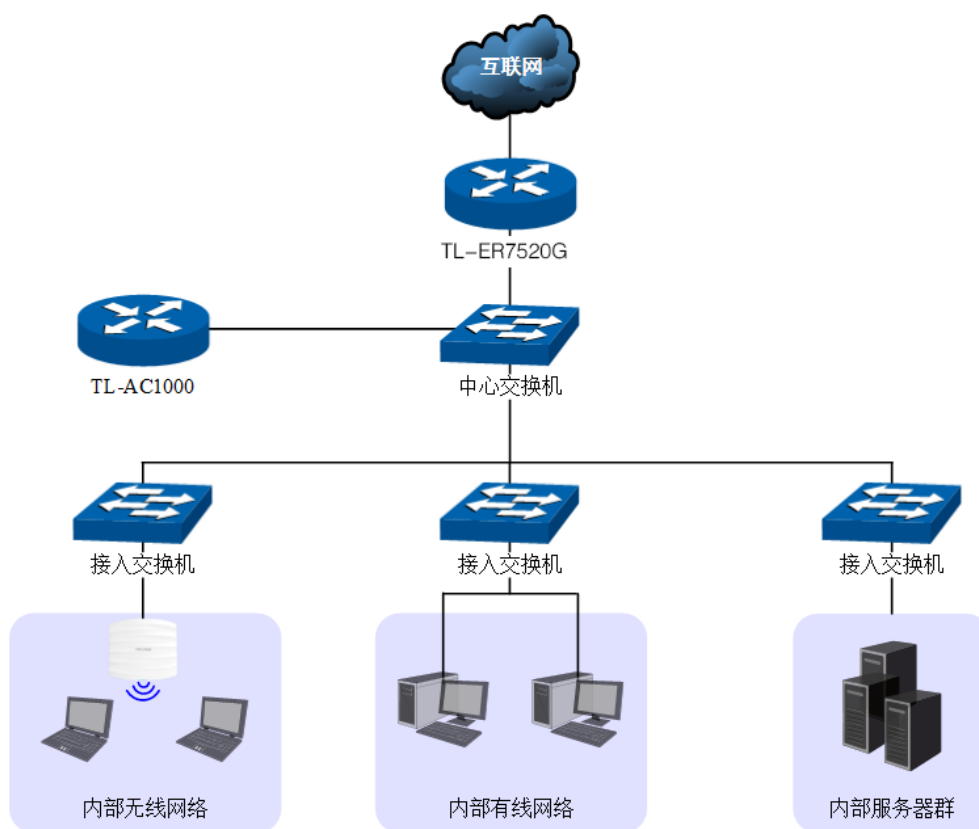
图 11-22 微信连Wi-Fi应用拓扑图
