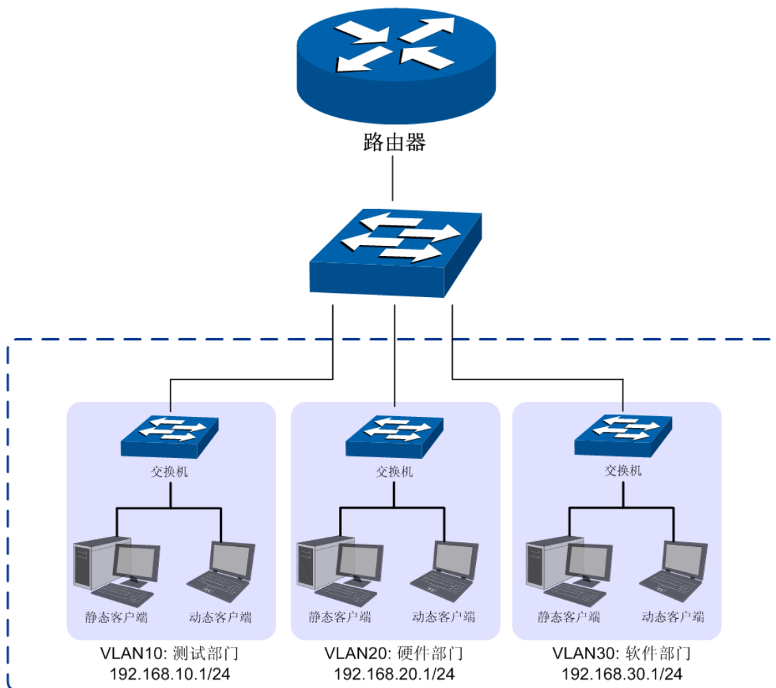
图 3-17 DHCP服务器功能组网举例
