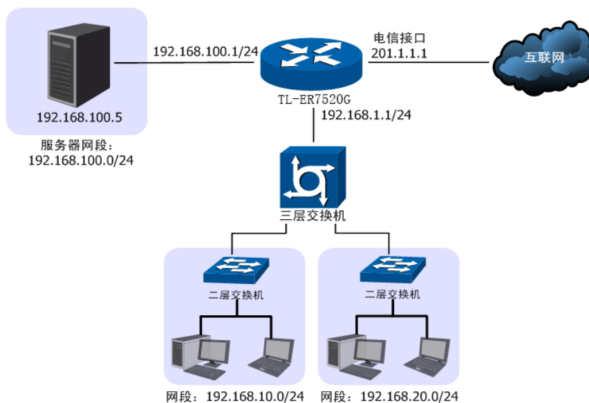
图 7-11 一对一NAT功能组网应用
