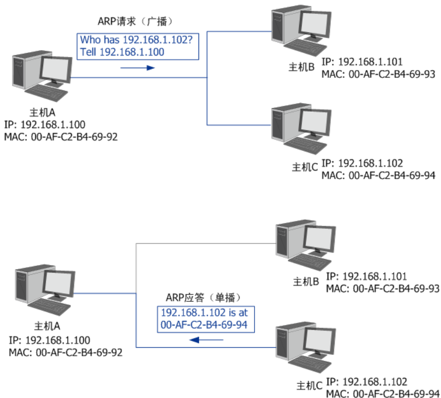
图 8-2 ARP解析过程
