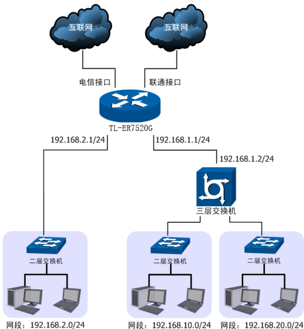
图 7-5 NAPT功能组网应用
