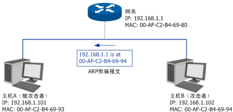
图 8-3 ARP欺骗-欺骗主机
