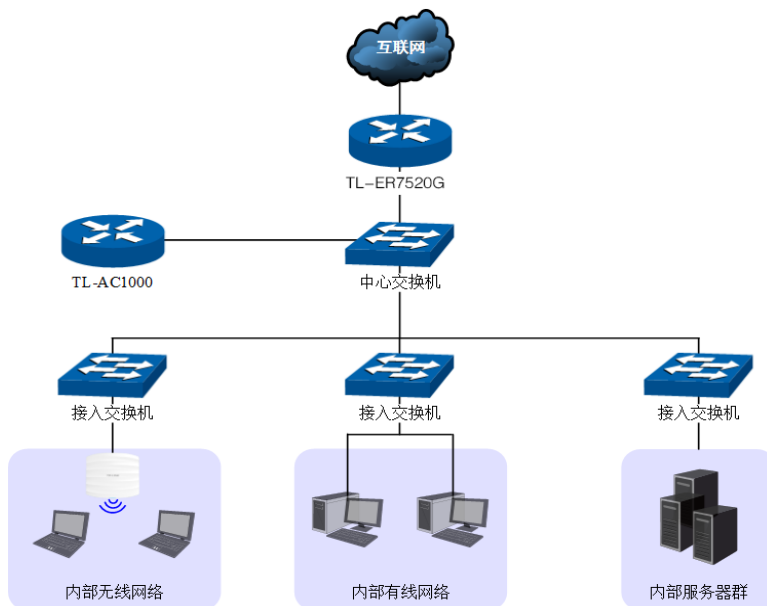
图 11-9 使用内置的Web服务器和认证服务器应用拓扑图
