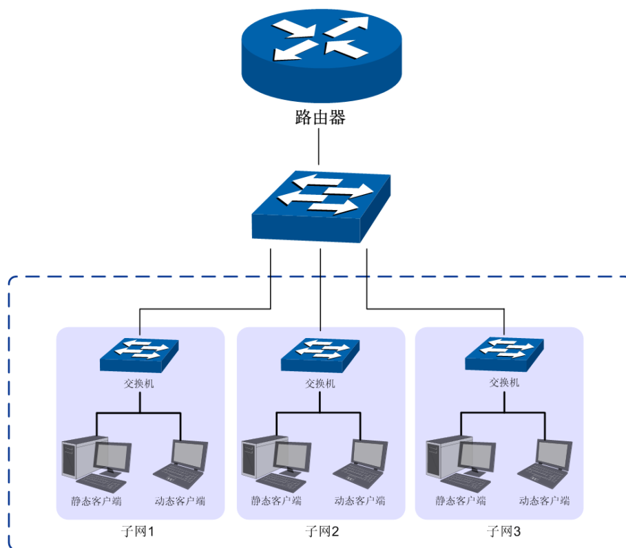
图 3-11 DHCP服务器功能应用环境
