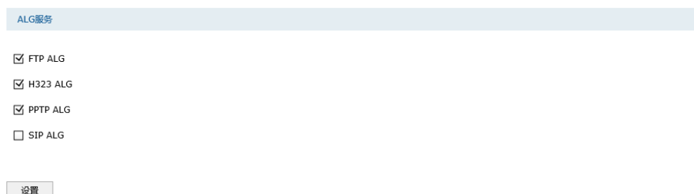
图 7-15 ALG服务界面-设置ALG服务
