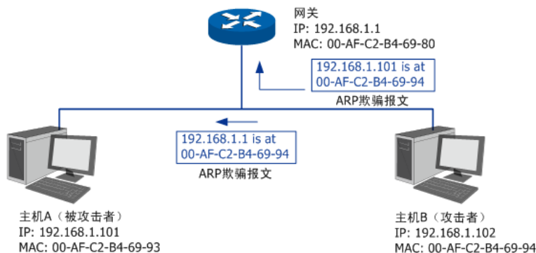
图 8-5 ARP欺骗-双向欺骗
