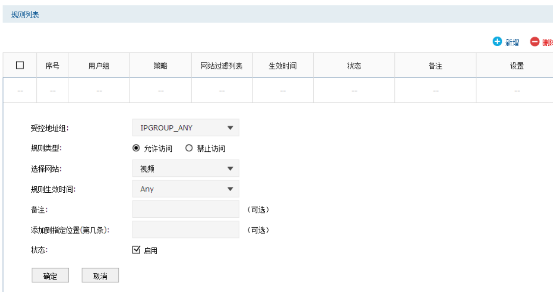
图 9-6 网站过滤规则设置界面
