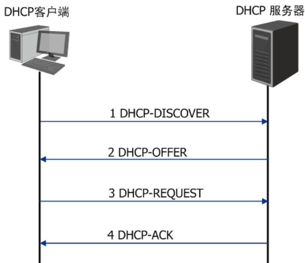
图 3-10 动态获取IP地址的过程
