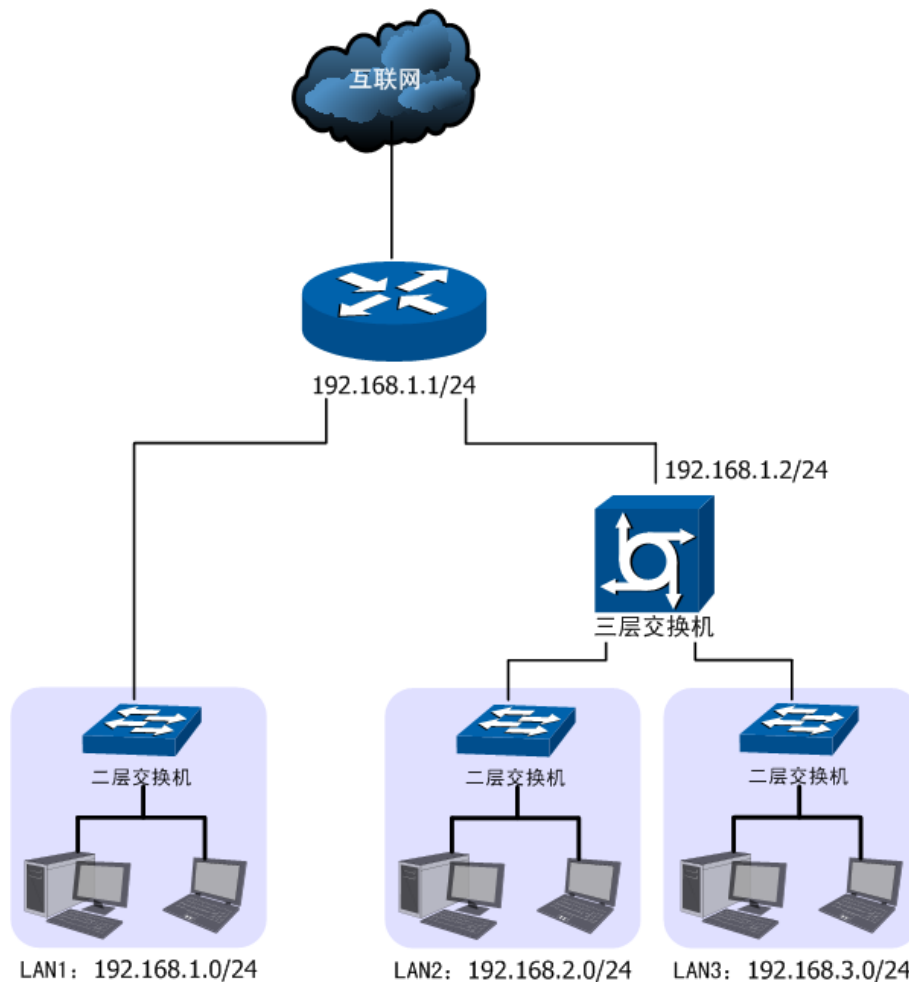
图 7-41 静态路由功能组网应用
