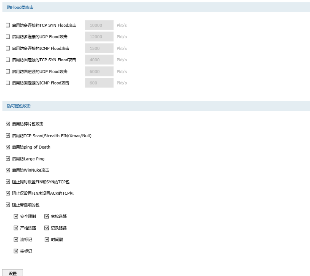
图 8-11 攻击防护设置界面
